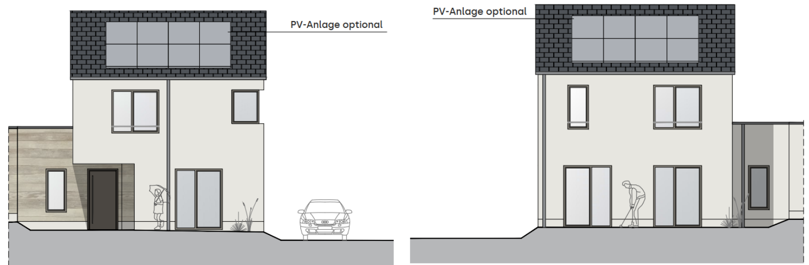
Ansicht 3 (Gartenseite)
