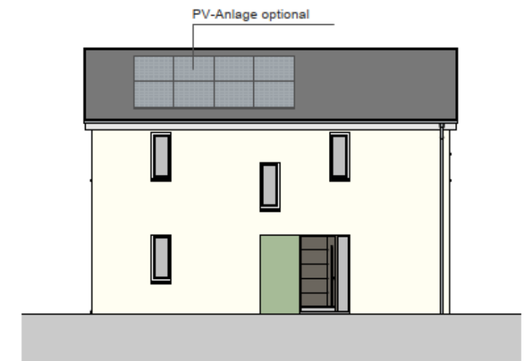
Ansicht 2
