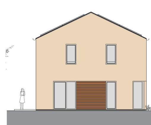
Ansicht 3
