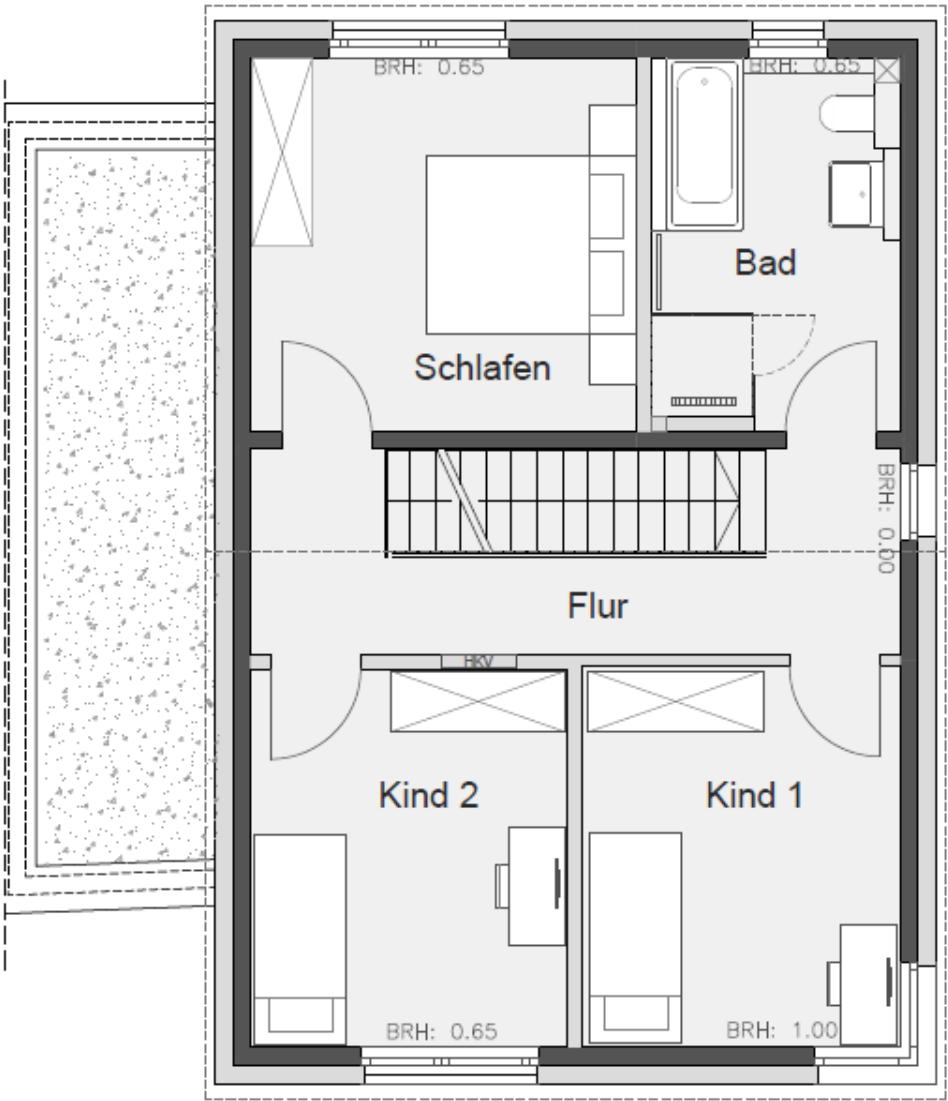
Obergeschoss
