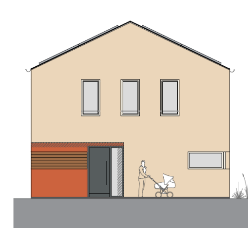
Ansicht 1
