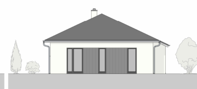
Ansicht 2
