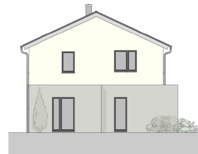
Ansicht 4
