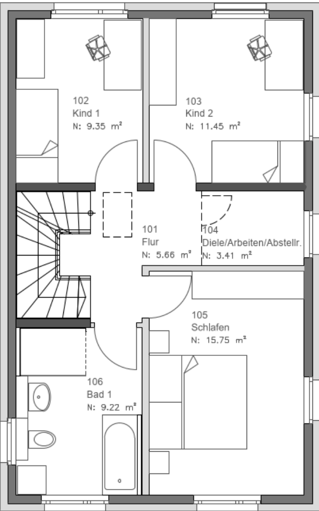
Obergeschoss
