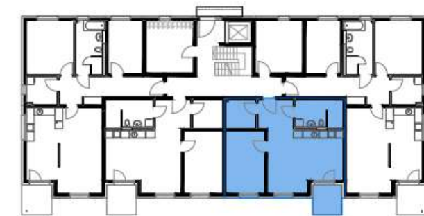
Erdgeschoss:
